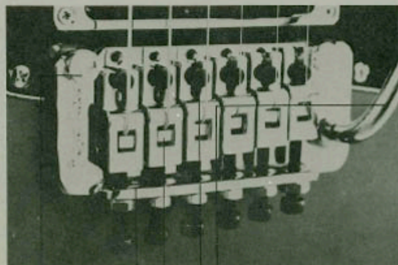
先端リアクションを可能にしたアイフロック。 このプレートをはじめ、他のパーツに調整性を確保した構造が入れられている。 真鍮のメッキで弦をガンナリとキープ。
